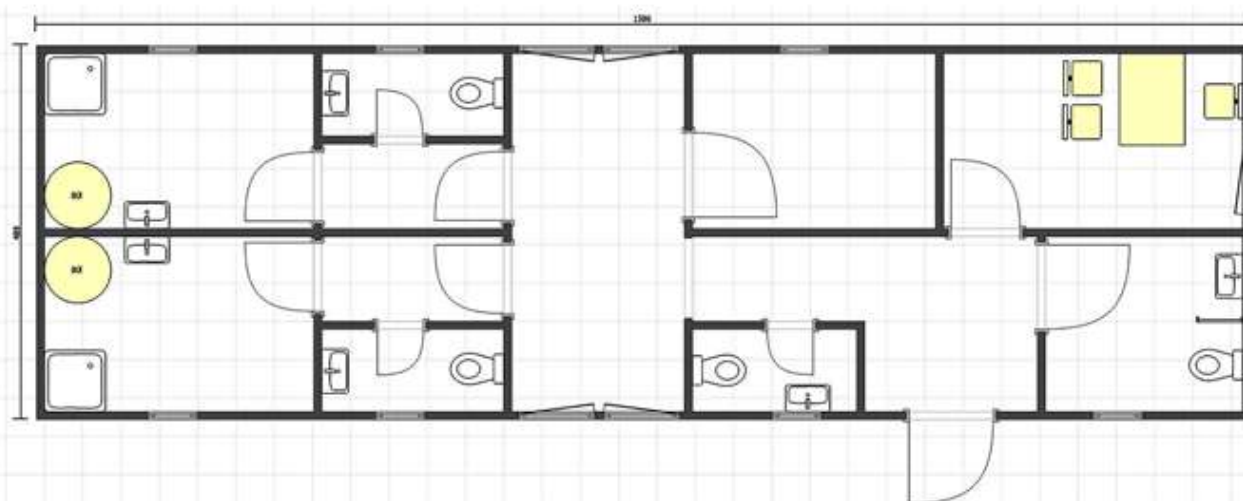
ÉTKEZŐVEL ÉS SZANITEREGYSÉGGEL ELLÁTOTT IRODAÉPÜLET
