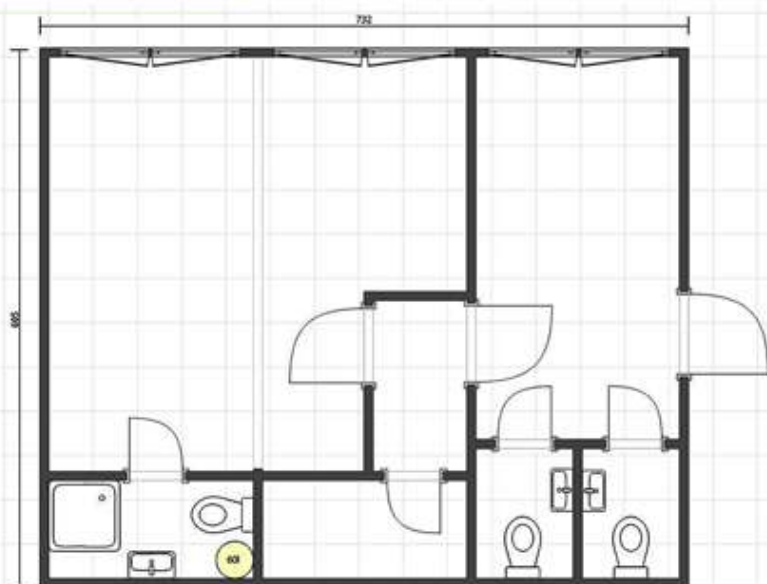
ZUHANYZÓVAL ÉS HÁROM WC-VEL ELLÁTOTT IRODAÉPÜLET
